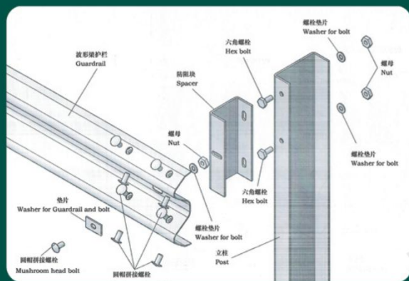
安装分解图/Installation Decomposition Diagram
